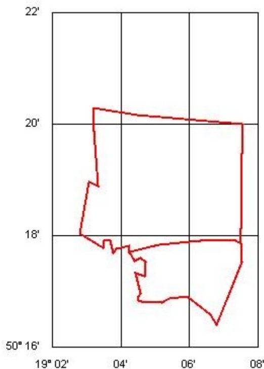
Rysunek1-1. Lokalizacja obszarów górniczych „Czeladź” i „Milowice” eksploatowanych przez KWK „Saturn”
